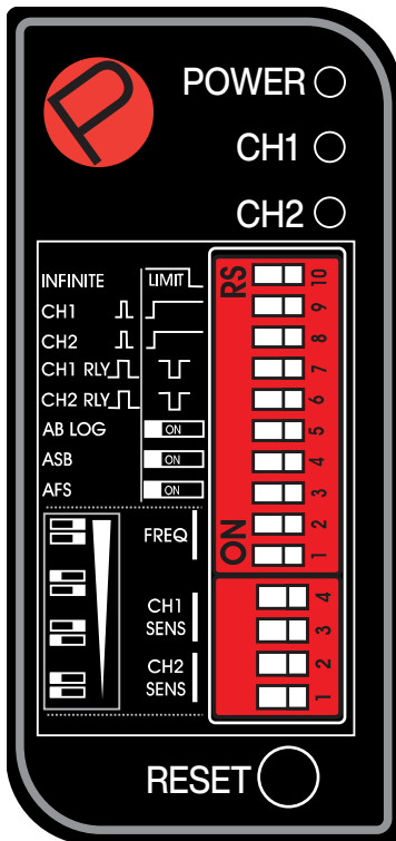
Bild3. LC20-2 Frontansicht
